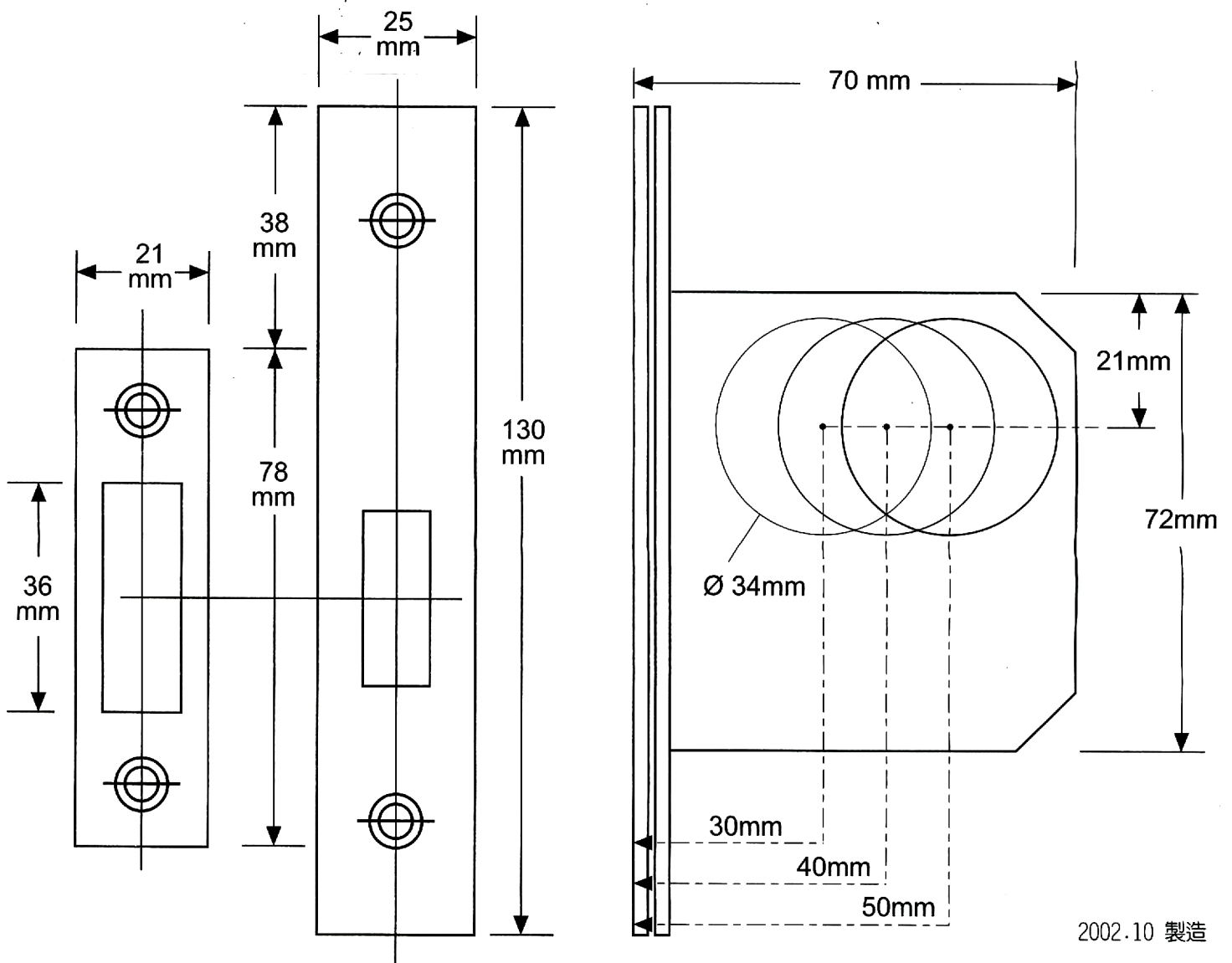
尺寸圖
