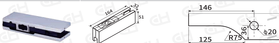
CH-200 上夾角(砂/亮)
