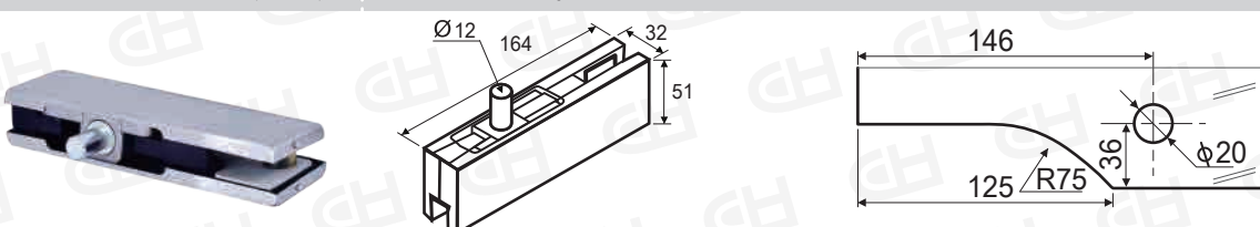
CH-400 L型夾角(砂/亮)
