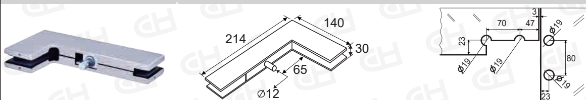
CH-800 ST鎖夾
