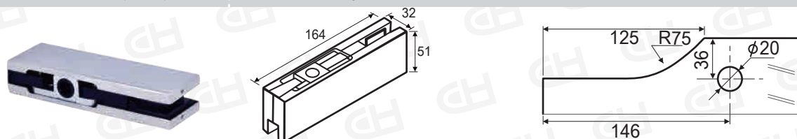
CH-300 一字型夾角(砂/亮)
