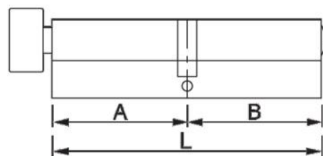
葉片伸縮鎖匙
