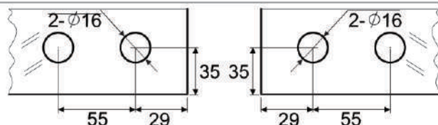
折疊門下包角 (雙) CH-8700A-I3
