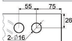
折疊門上包角 (雙) CH-8700A-IO
