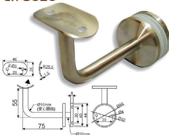
玻璃扶手管座
