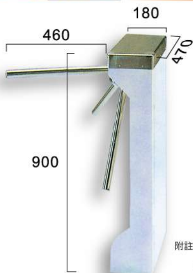
單向門(烤漆)
