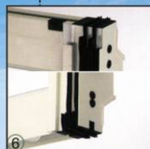
⑥ 專利設計大鉤上下端L型雙層式氣密結構，氣密隔音超強。
